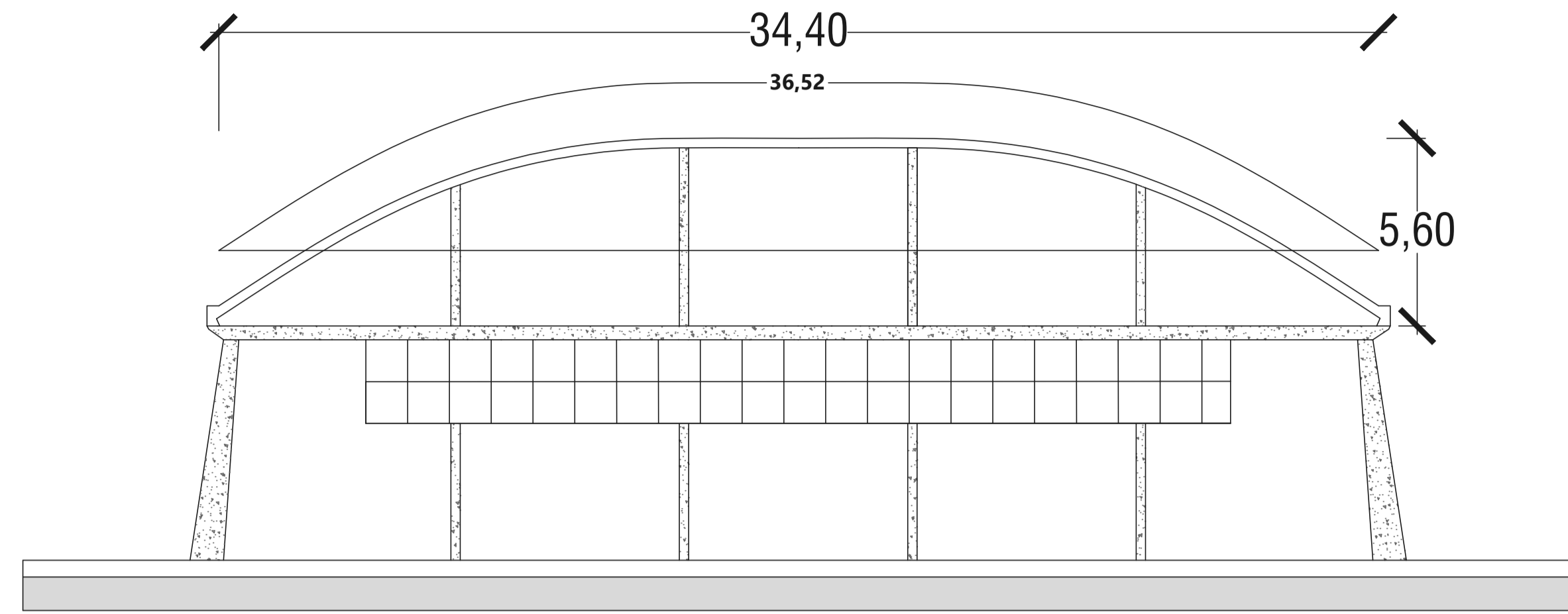
2 ELEVÇÃO FRONTAL
