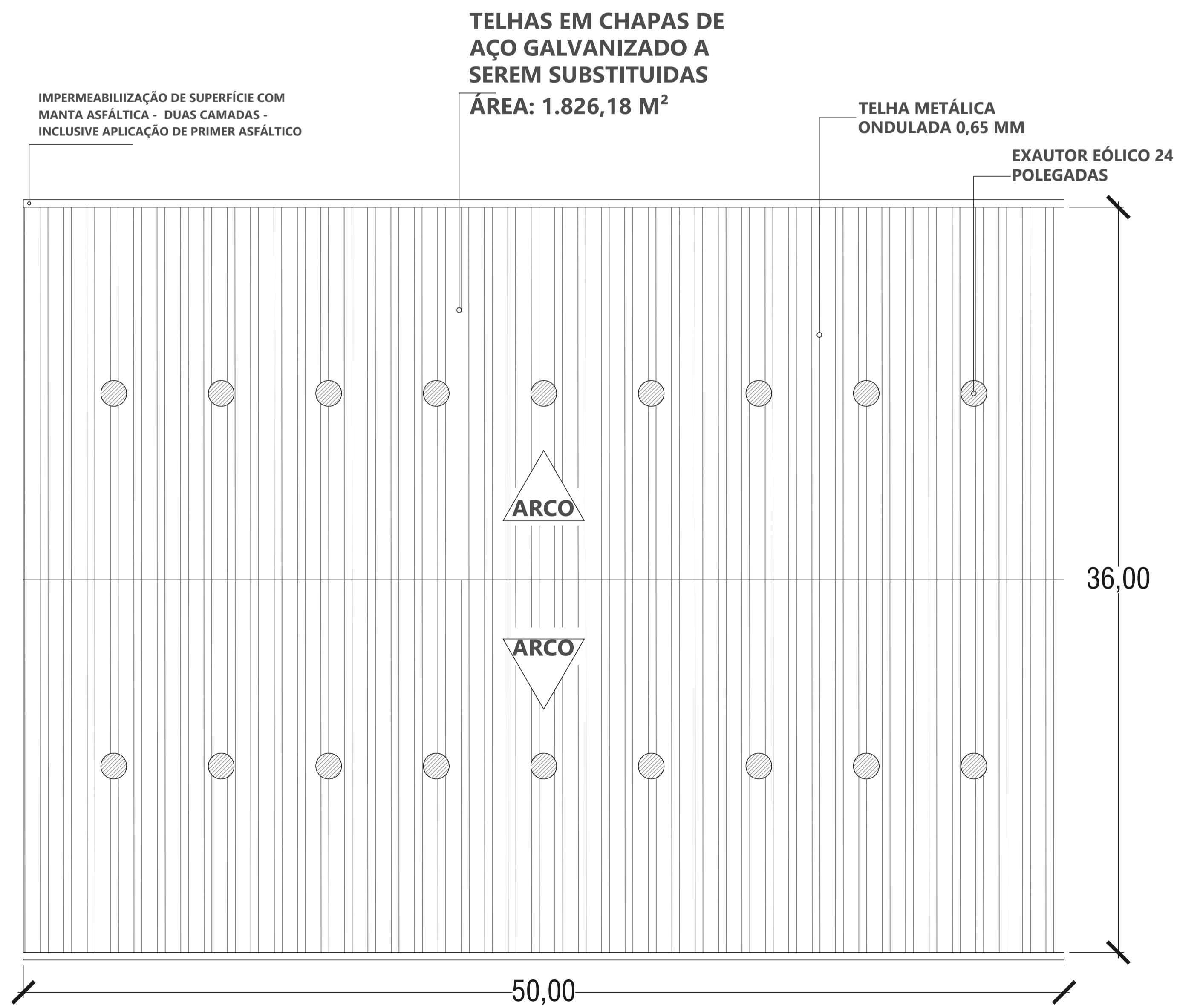
1 PLANTA DE COBERTURA
